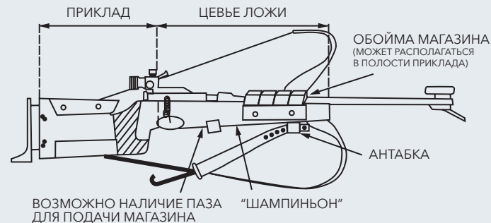
■ РИСУНОК 1 СХЕМА БИАТЛОННОЙ ВИНТОВКИ
