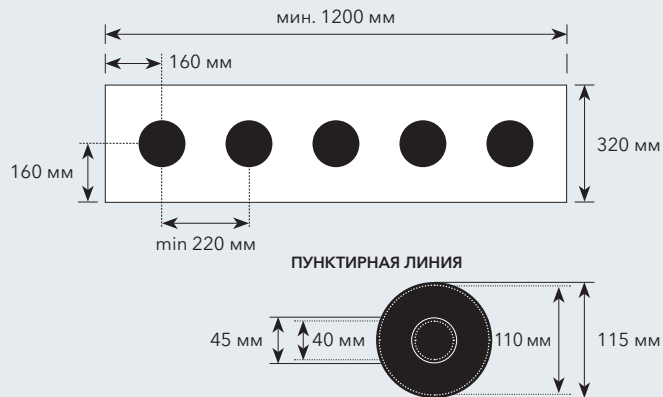
РИСУНОК 3 СТАНДАРТНЫЕ РАЗМЕРЫ БУМАЖНЫХ МИШЕНЕЙ
