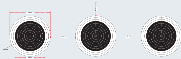
РИСУНОК 3А БУМАЖНЫЕ МИШЕНИ С КРУГАМИ
