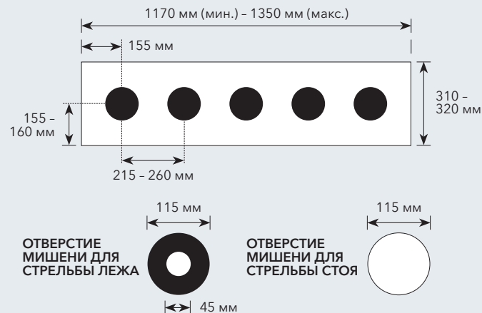
■ РИСУНОК 2 СТАНДАРТНЫЕ РАЗМЕРЫ МЕТАЛЛИЧЕСКИХ МИШЕНЕЙ
