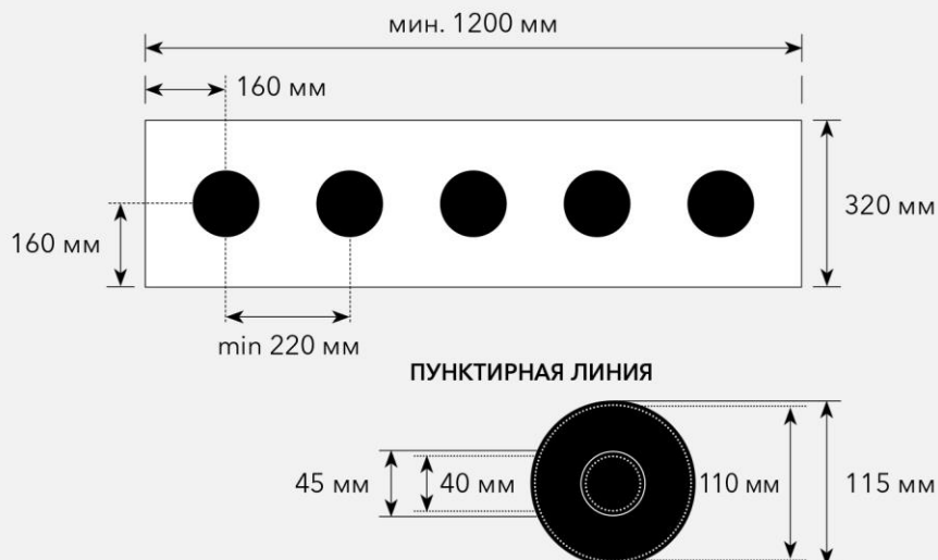
■ РИСУНОК 3 СТАНДАРТНЫЕ РАЗМЕРЫ БУМАЖНЫХ МИШЕНЕЙ
