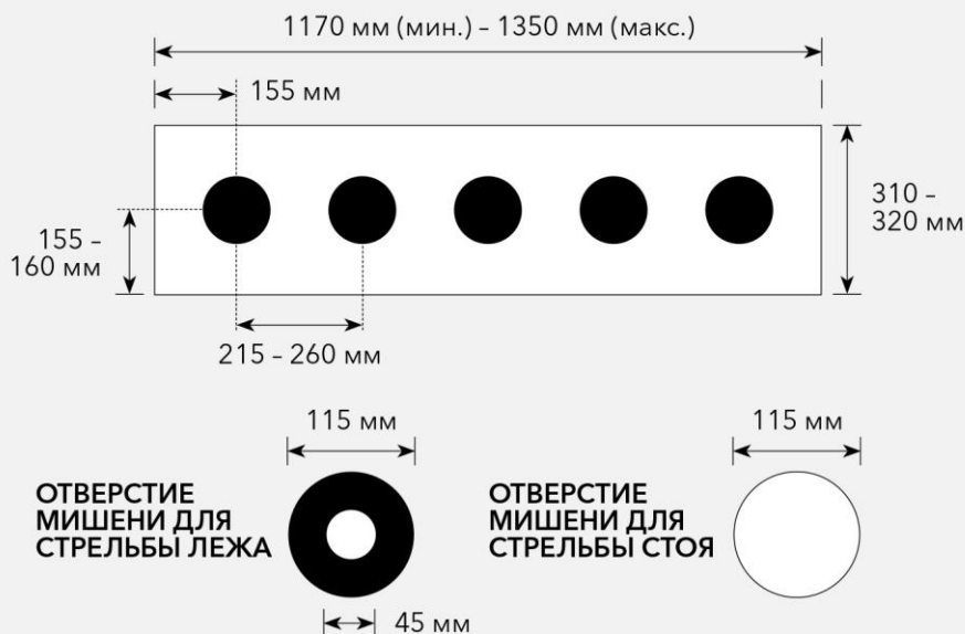
■ РИСУНОК 2 СТАНДАРТНЫЕ РАЗМЕРЫ МЕТАЛЛИЧЕСКИХ МИШЕНЕЙ
